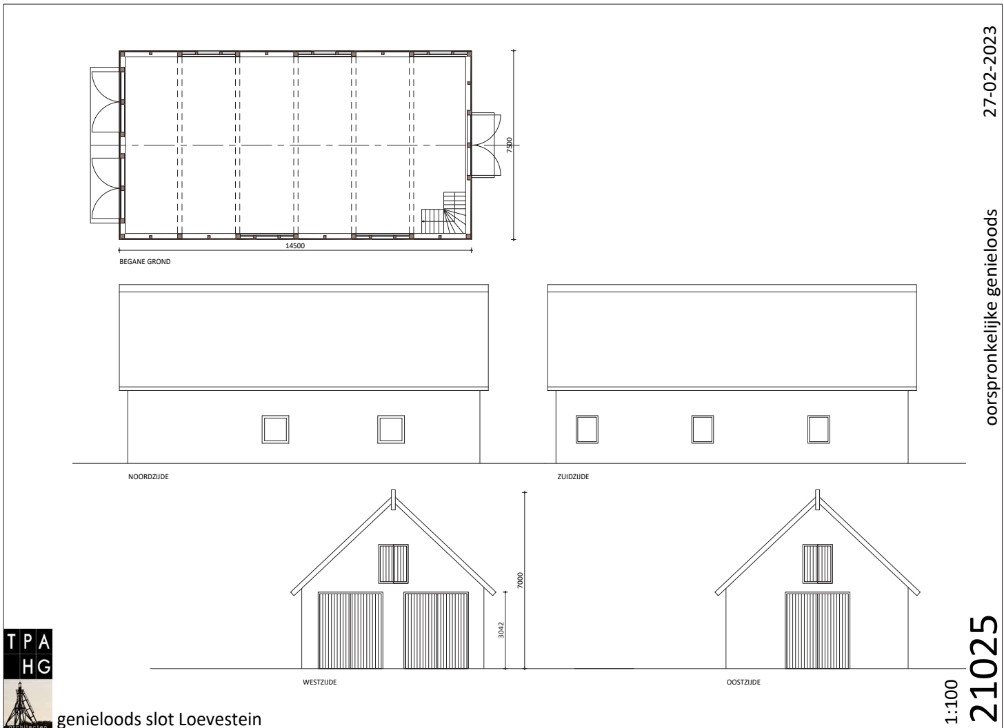
globale uitwerking oorspronkelijke genieloods
