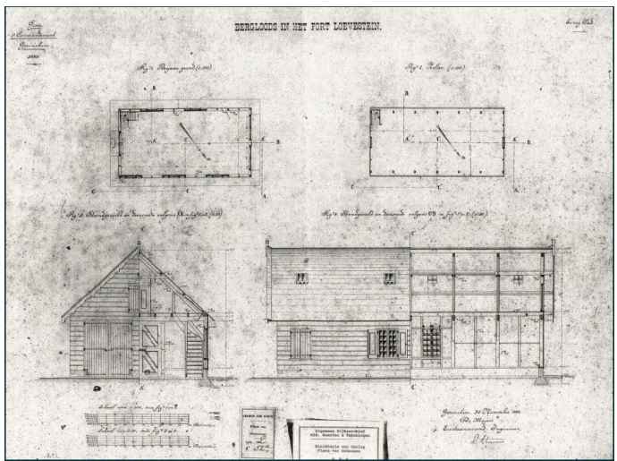
Rechts de oude bouwtekeningen van de oorspronkelijke loods, met uitvergrotingen van de zijgevel aan de kant van het slot en de zuidgevel. Linksboven een foto van de barak met een berghok aan de zijkant. Door de rode en gele lijn kunnen we de uiteindelijke afmeting en plaats inschatten.
